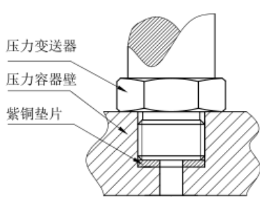
螺纹前端面密封安装图
