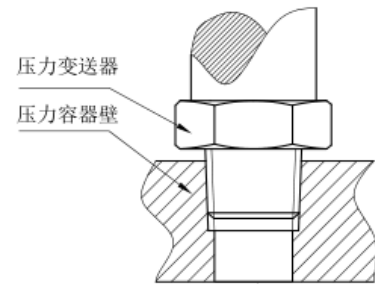
锥度螺纹密封安装图
