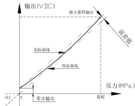
电压输出曲线图
