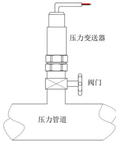
正确安装方式：垂直安装
