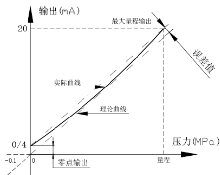
电流输出曲线图
