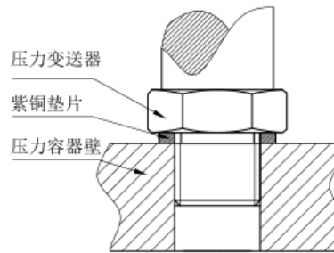
六角端面密封安装图
