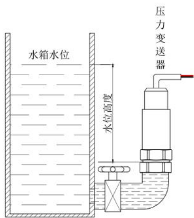
正确水位测量
