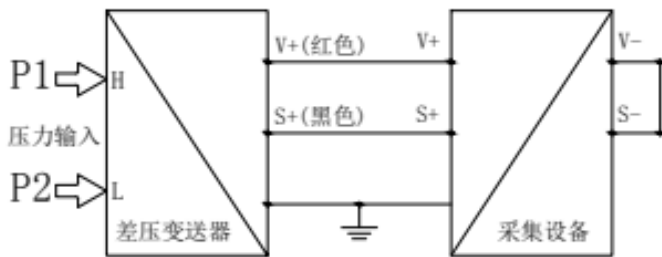
4-20mA电流输出接线图
